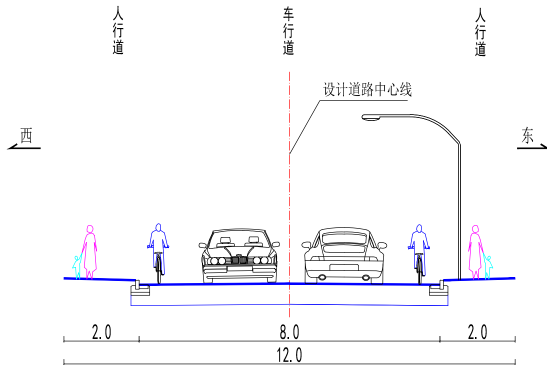
安轩路 (华铁路-16-04地块) 道路标准横断面
